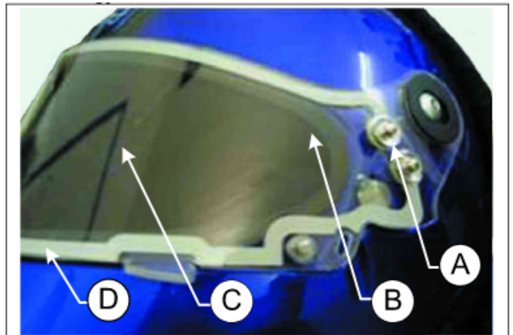
图1: 头盔透明电热片图解
